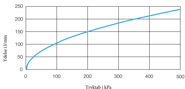
Ydelses-diagram
